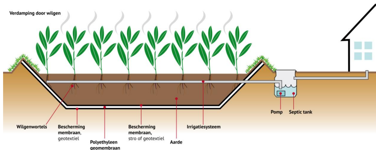
Figuur 1. Schematische weergave van een wilgenzuivering (illustratie: Gebca Velema, Probos).
